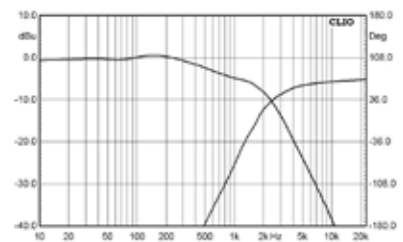
Sistema 20.50 - Risposta elettrica
