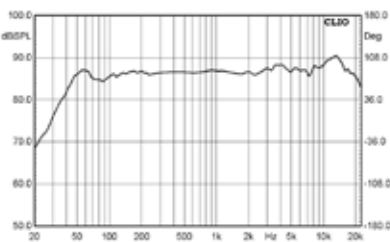
Sistema 20.50 - Risposta in frequenza
