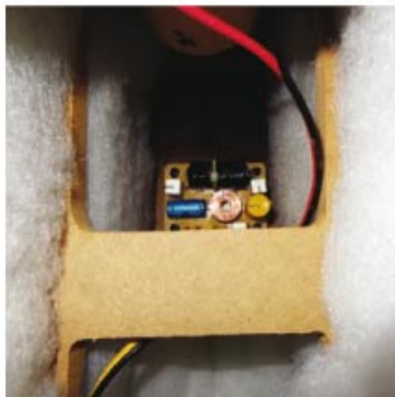
Tesi 260:n jakosuodin on basson osalta ensimmäistä astetta (6 dB/oktaavi). Elektrolyyttikondensaattori ja vastus tasaavat elementin impedanssia.
